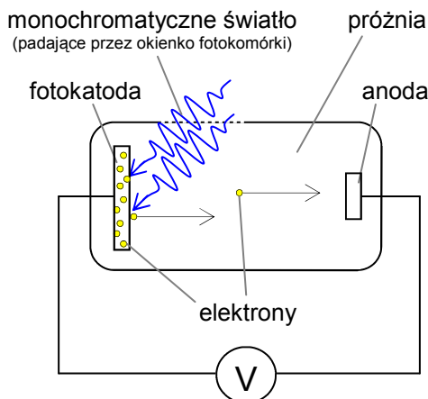
Rys. 1. Schemat ideowy aparatury do badania efektu fotoelektrycznego
