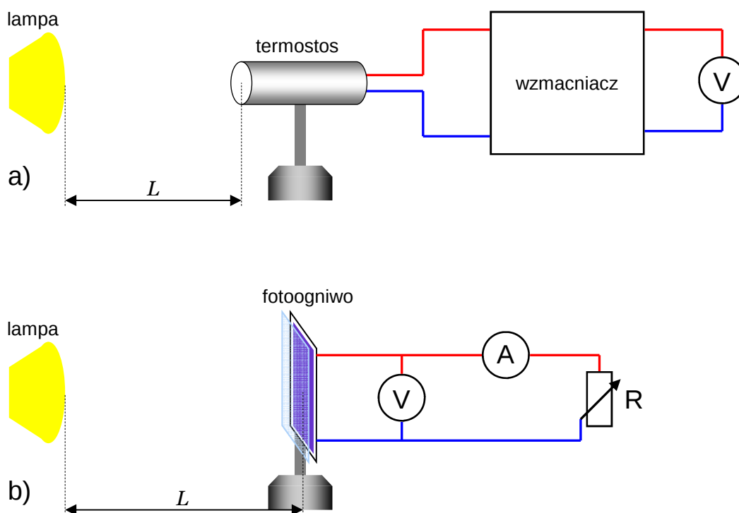
Rys. 2. Schemat ideowy aparatury do badania efektu fotoelektrycznego wewnętrznego a) układ z termostosem, b) układ z fotoogniwem
